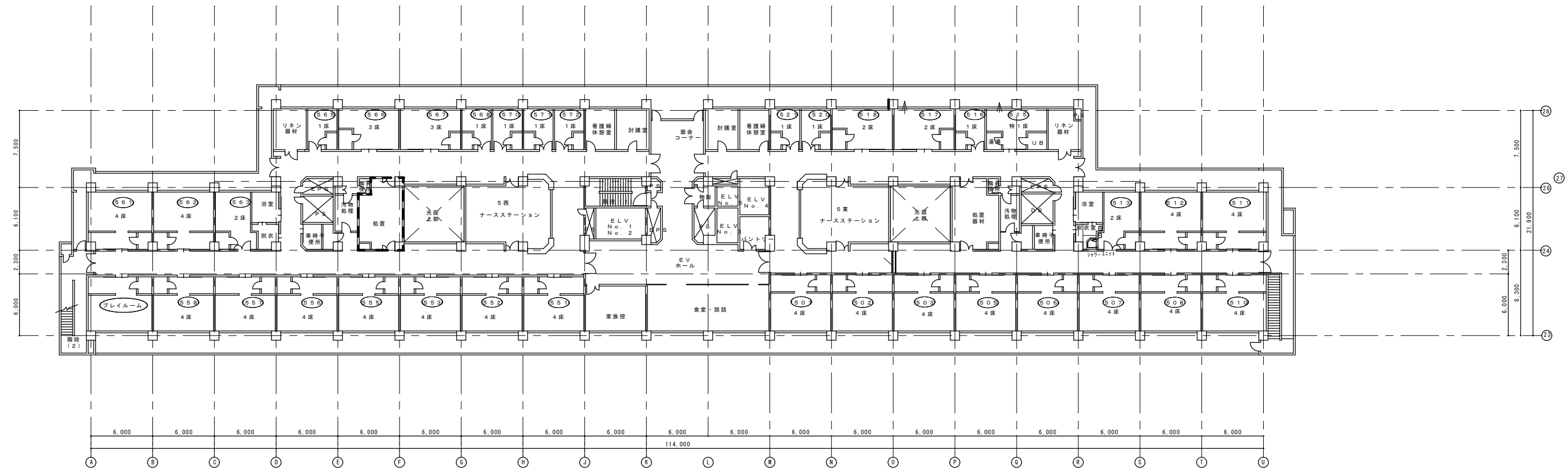
5階平面図
